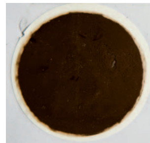
Filterpads mit Standard-Heizöl
